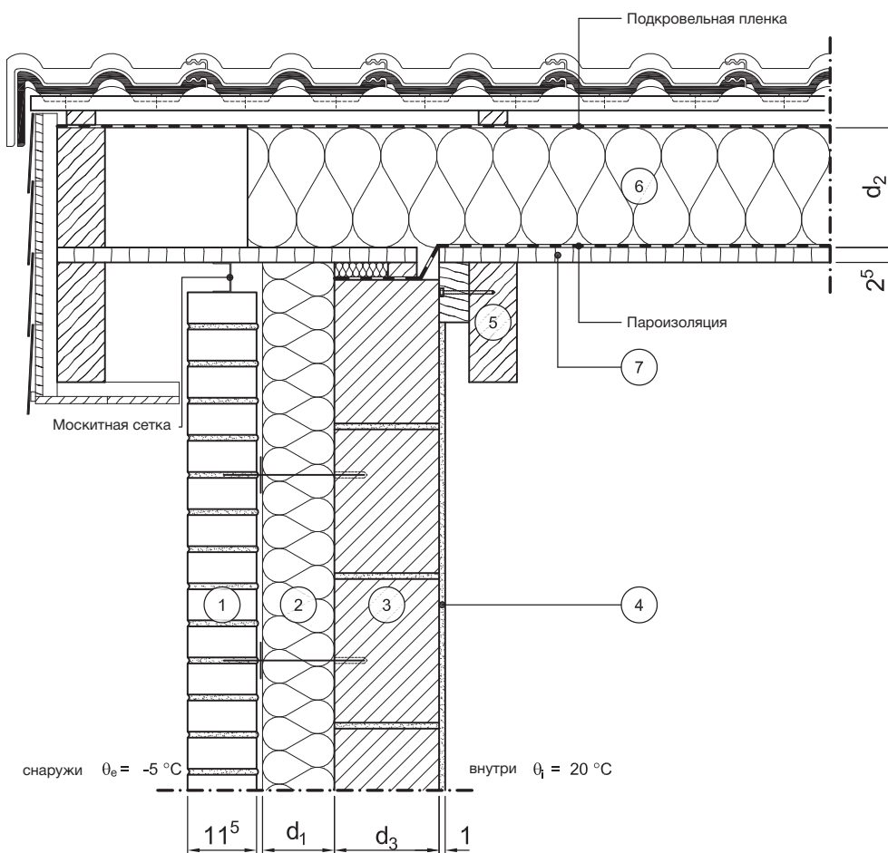
Вертикальный разрез
