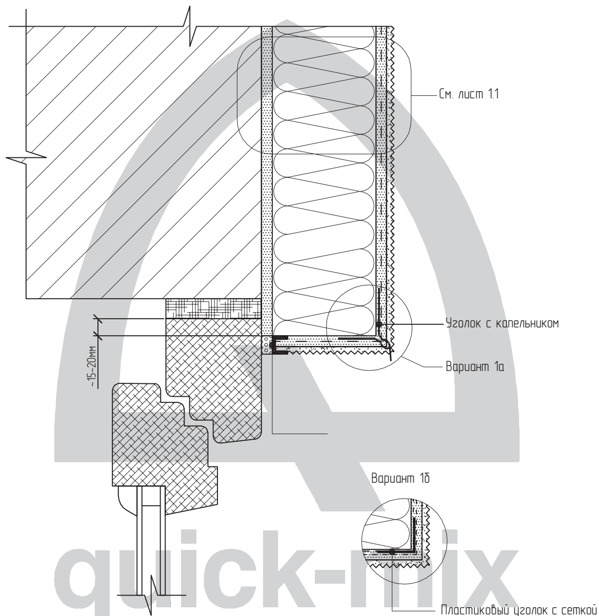
Вертикальный разрез
