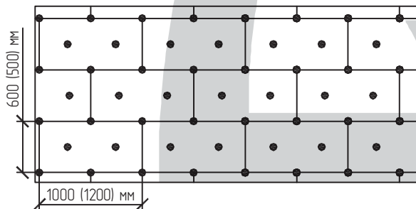
Схема дюбелирования 8,3 дюб./м²
