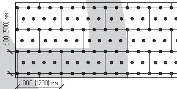
Схема дюбелирования 13,3 дюб./м²
