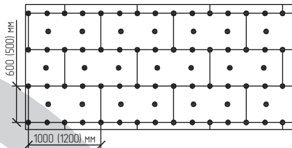
Схема дюбелирования 11,7 дюб./м²
