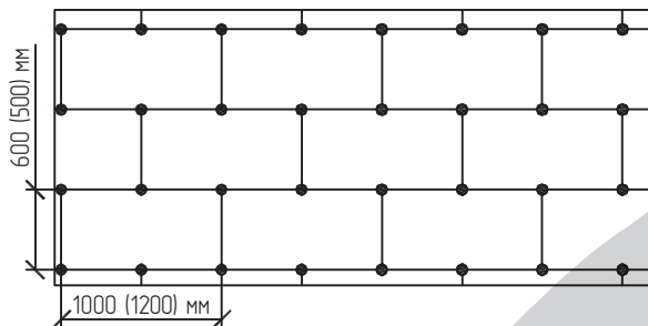
Схема дюбелирования 5 дюб./м²
